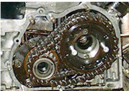
Kæde og kædehjul meget slidte, ca 15 mm nedhæng, udskiftet, den gamle kæde er hængt udenpå den nye.
