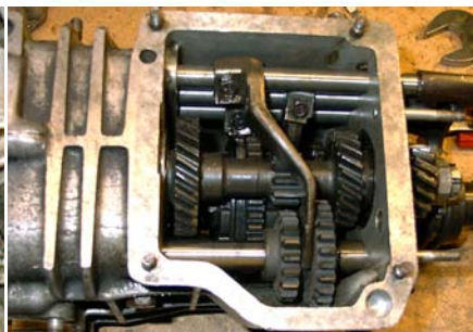
Gearkassen renoveret, monteret nye tandhjul for 1. og baggear.
